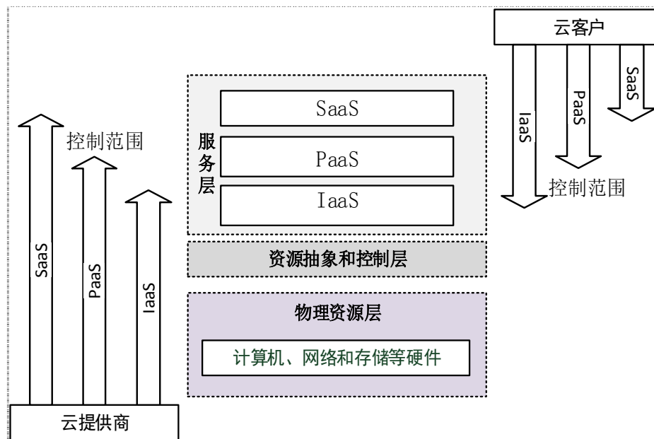
图 4-1 云计算服务模式与控制范围的关系
